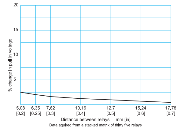
Fig. #8 Alternate Pairs Matrix.
