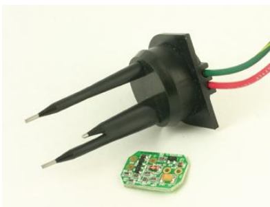
洗涤液电导传感器
