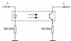
試験回路
