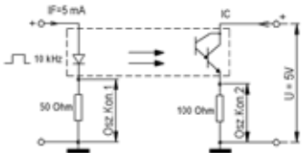
試験回路
